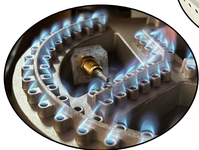
Quemador de Ø 180mm y Termocupla de Seguridad
